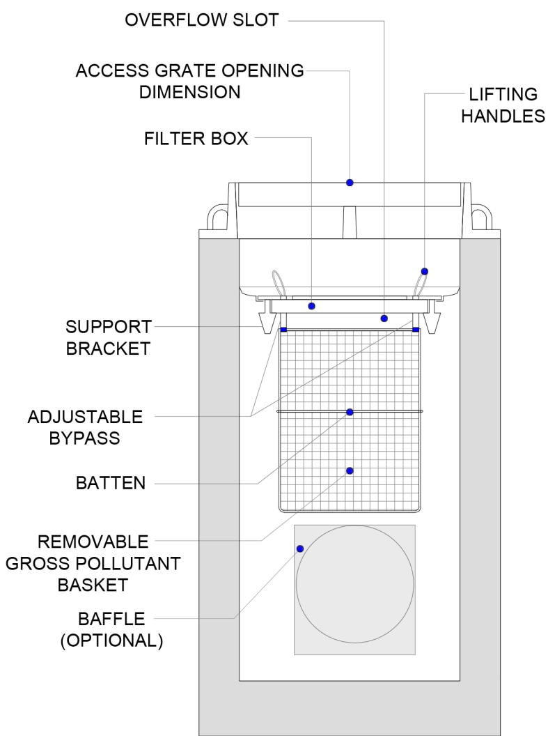
SECTION A-A
